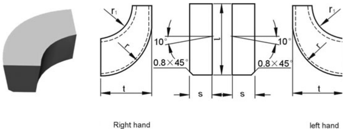
Tungsten carbide brazed tips type B3
