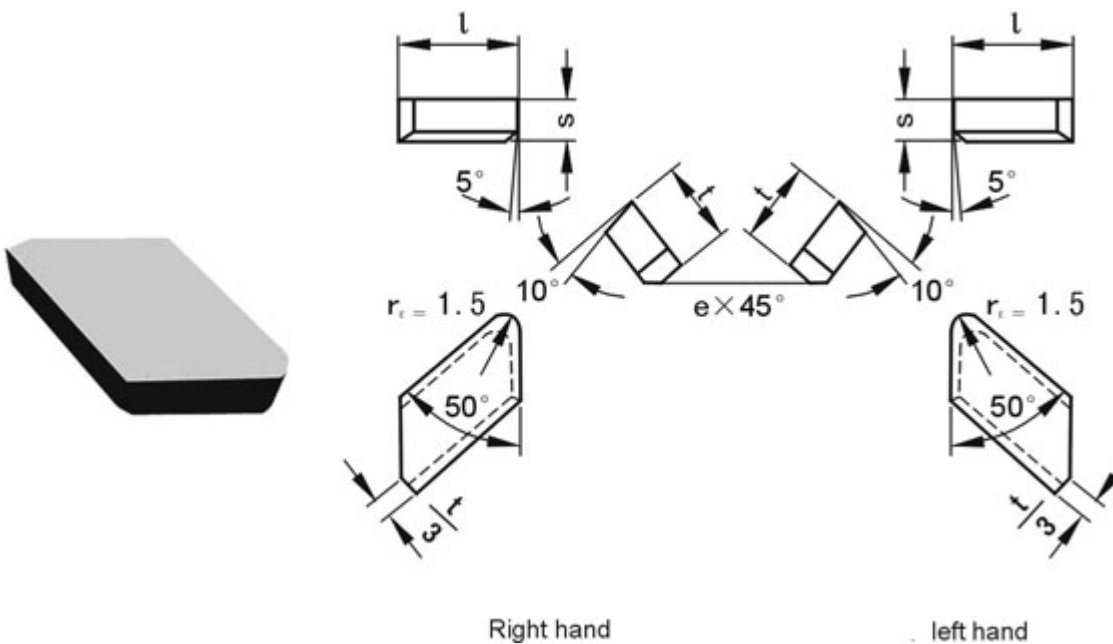
Tungsten carbide brazed tips type B1
