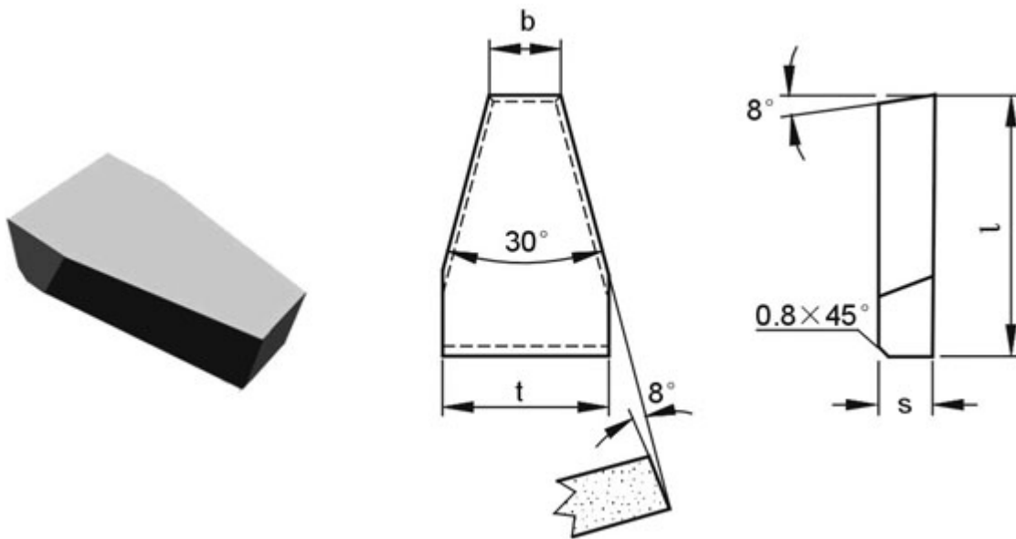
Tungsten carbide brazed tips type C2
